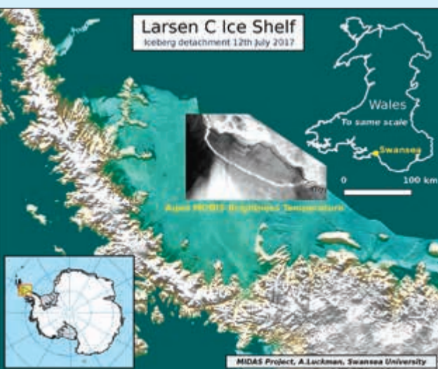
صورة عبر الأقمار الاصطناعية تظهر جبل الجليد «إيه 68»، خلال انفصاله عن الجرف الجليدي لارسن سي
