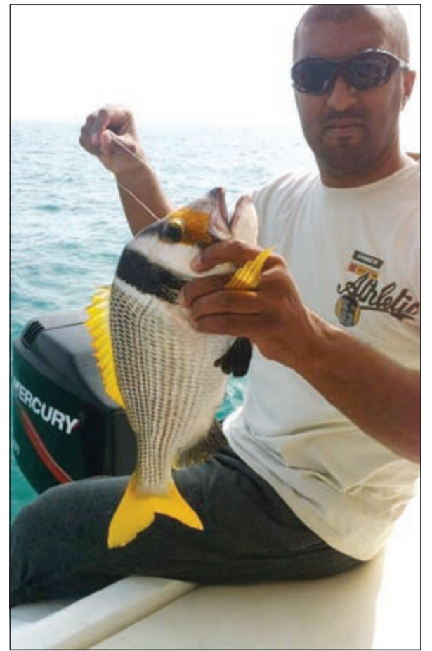
خوش فسكر
