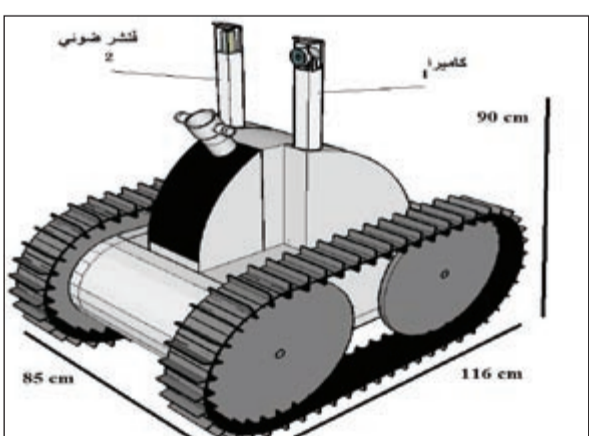
الروبوت المكافح للحرائق
