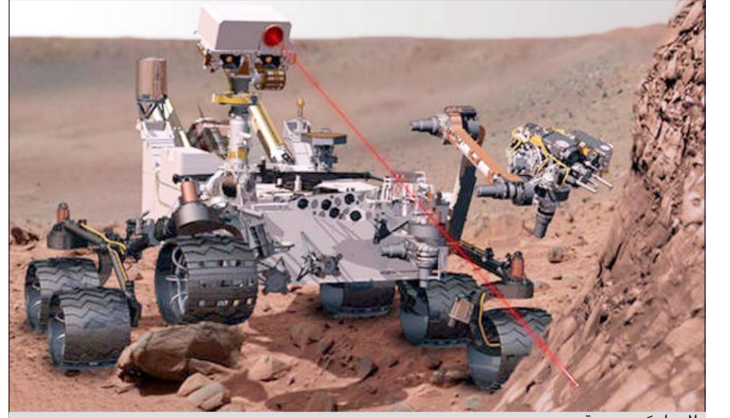
المسبار كوريوسيتي
